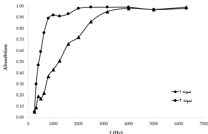
شکل ۴- ضریب جذب صوت نمونه‌های فرش دستباف (با مشخصات ساختاری مطابق جدول ۳) در لوله امپدانس (نگارنده، ۱۴۰۰)
