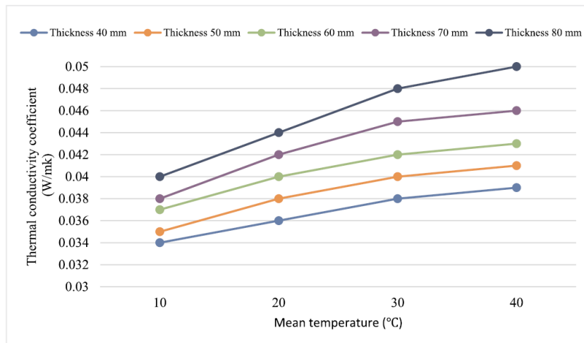
شکل ۱- تأثیر دما بر هدایت گرمایی الیاف پشم در ضخامت‌های مختلف (همان: ۲۵۲)
