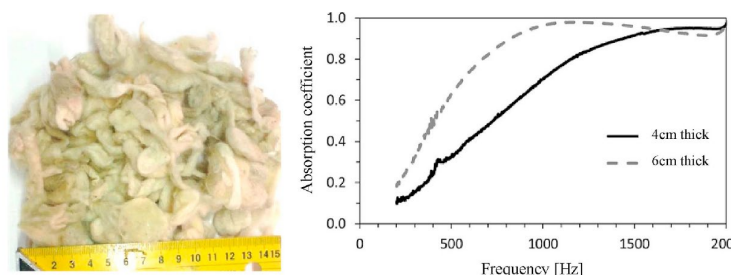
شکل ۲- ضریب جذب صوت پشم گوسفند (Islam & Bhat, 2019:11)
