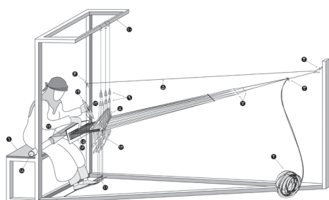
شکل ۴- تصویر شماتیک دستگاه تون‌بافی (نگارندگان، ۱۴۰۰)
